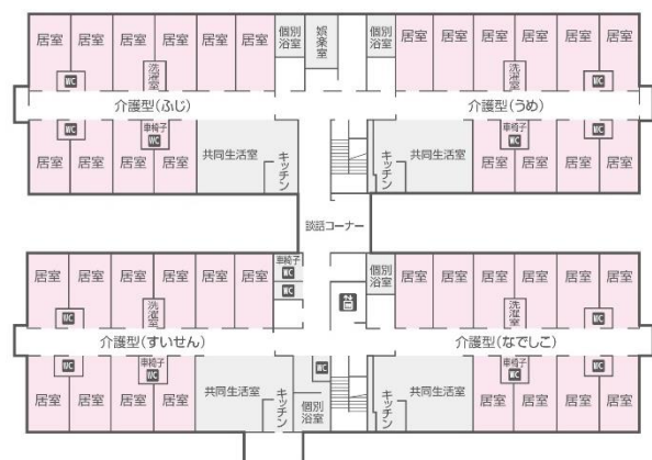
2F 平面図
